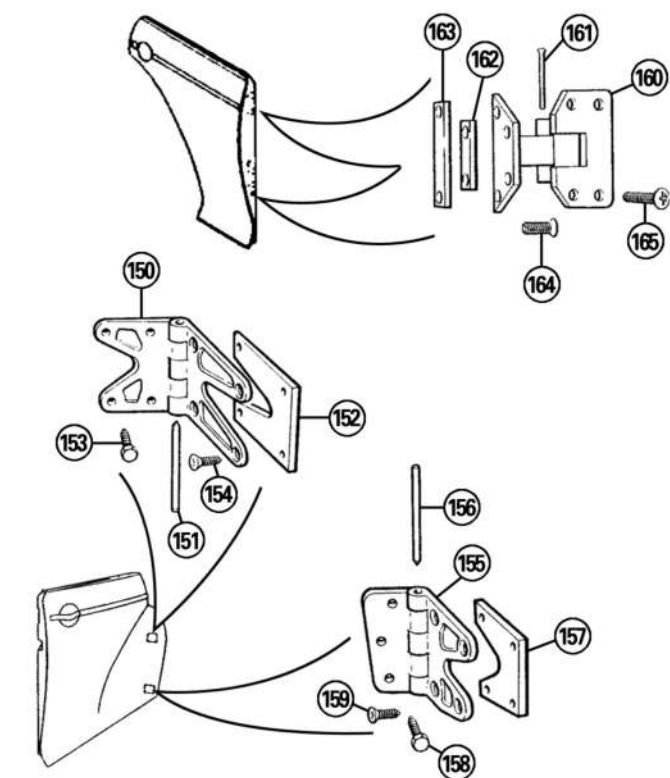
Hinges
