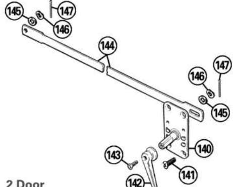
2 Door
